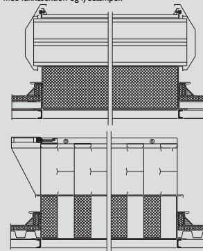
Detalje af Labyrinth MKI på monteringsramme, med lukkesektion og lyddæmper.
