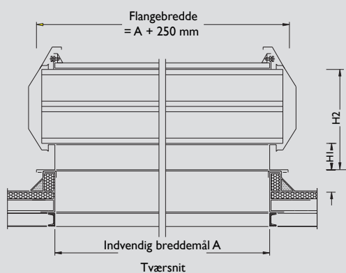
Detalje af Labyrinth MKI på monteringsramme, med lukkesektion.
