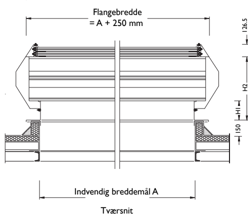
Detalje af Labyrinth MK2 på monteringsramme, med lukkesektion.
